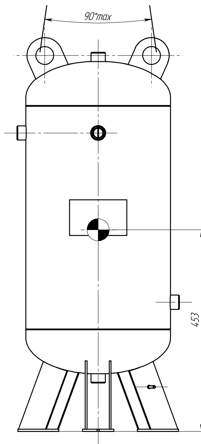
Схема строповки (1 : 5)
