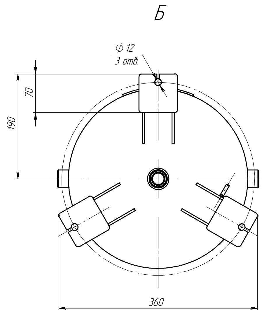
Схема строповки (1 : 5)
