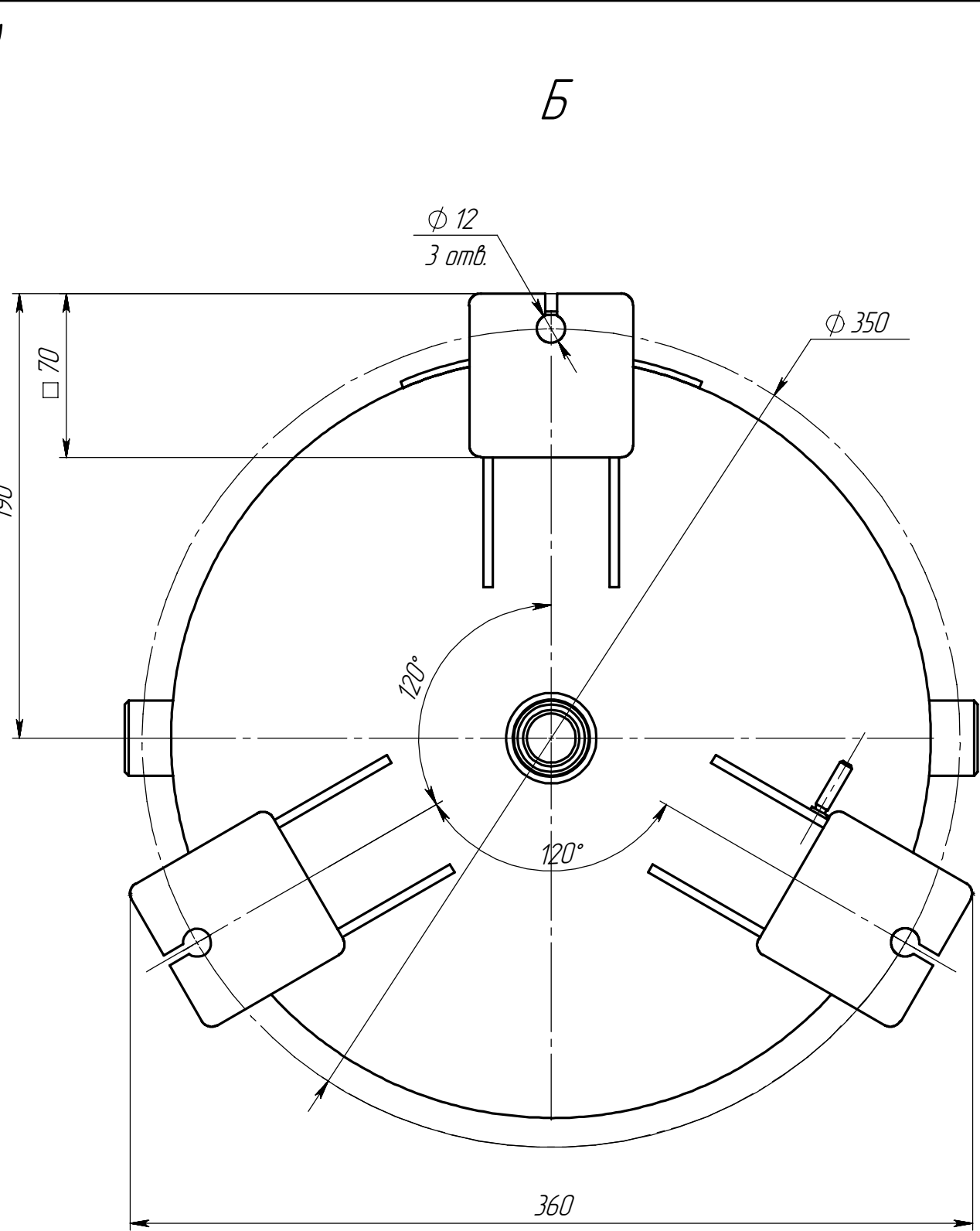
Схема строповки (1 : 5)
