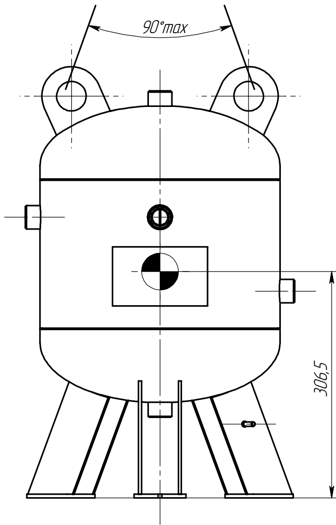
Схема строповки (1 : 5)
