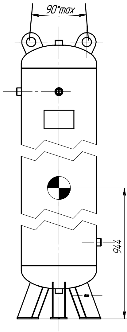
Схема строповки (1 : 10)
