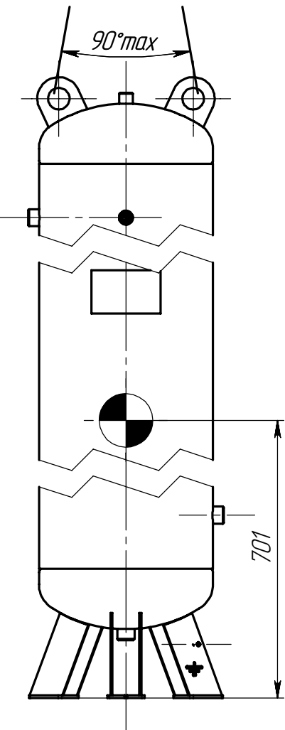
Схема строповки (1 : 10)
