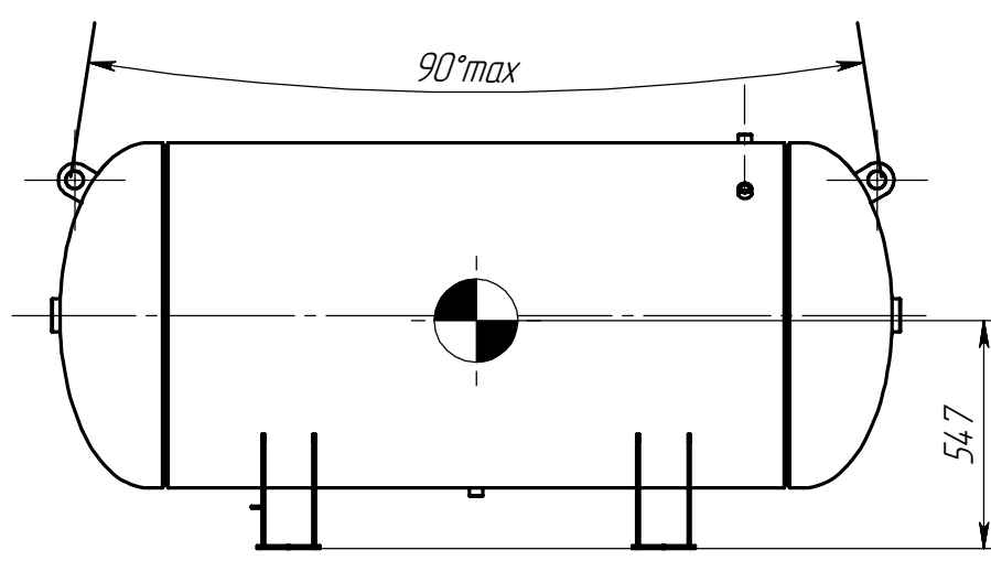
Схема строповки (1 : 20)
