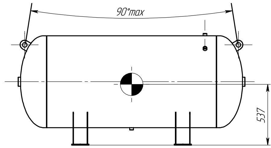
Схема строповки (1 : 20)
