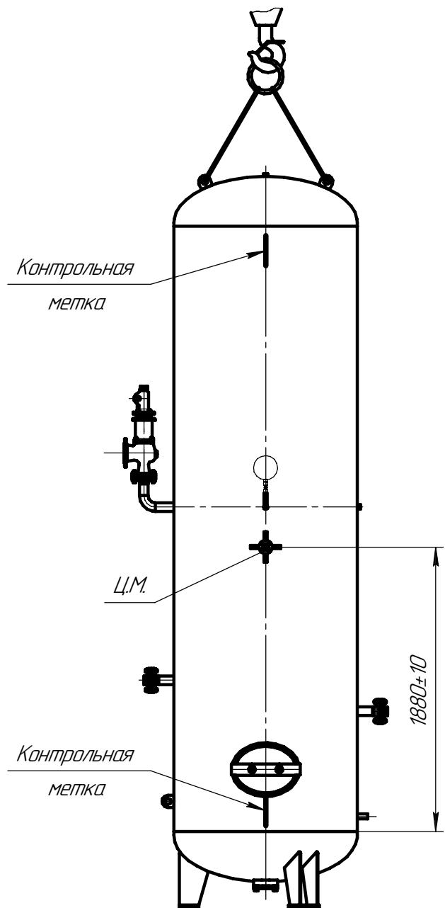
Схема строповки аппарата в вертикальном положении
