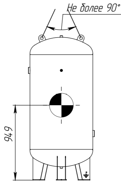
Схема strapовки аппарата в вертикальном положении
