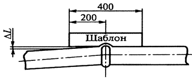
Рисунок 11. Схема определения отклонения от прямолинейности оси трубы
