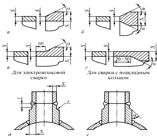
Рисунок 14. Стыковка элементов разной толщины
