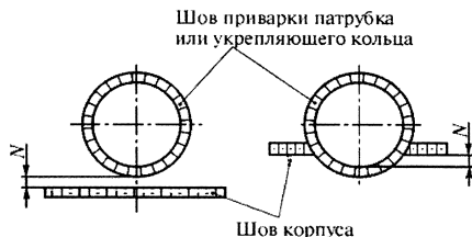
Рисунок 9. Схема определения расстояния между краем шва корпуса и краем шва приварки детали
