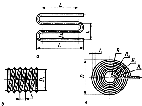
Рисунок 12. Размеры гнутых змеевиков
