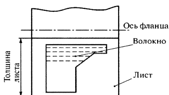
Рисунок 8. Схема вальцовки фланца приварного встык по плоскости листа
