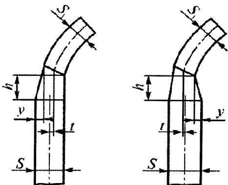
Рисунок 2 Узел соединения днища с обечайкой
