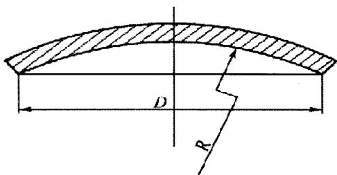
Рисунок 3. Сферическое неотбортованное днище
