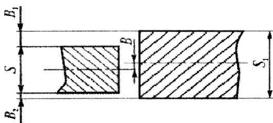
Рисунок 15. Смещение кромок
