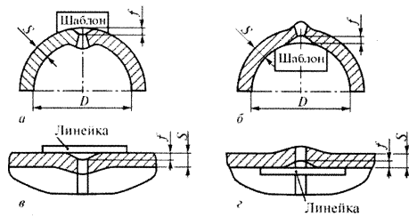
Рисунок 16. Контроль увода кромок продольных и кольцевых сварных соединений
