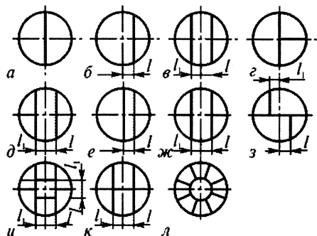
Рисунок 1. Расположение сварных швов заготовок выпуклых днищ
