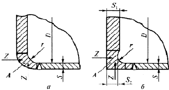
Рисунок 4. Плоские днища
