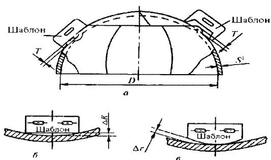
Рисунок 7. Отклонение формы полусферического днища
