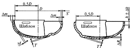
Рисунок 6. Отклонение размеров и формы эллиптического днища
