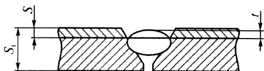
Рисунок 17. Усиление переходного шва в сварных соединениях двухслойных сталей
