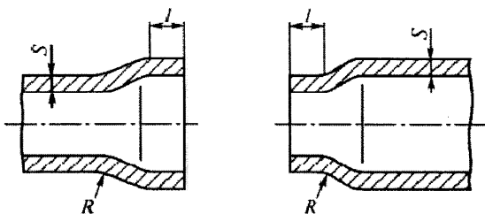
Рисунок 5. Отбортованный и переходный элемент
