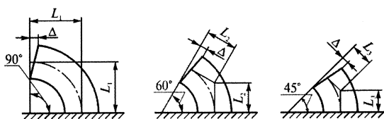
Рисунок 13. Схема определения размеров L_1 , L_2 , L_3 , \Delta отводов в зависимости от углагиба
